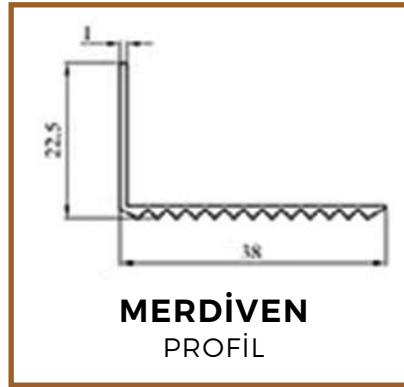
MERDİVEN BURUN PROFİL
